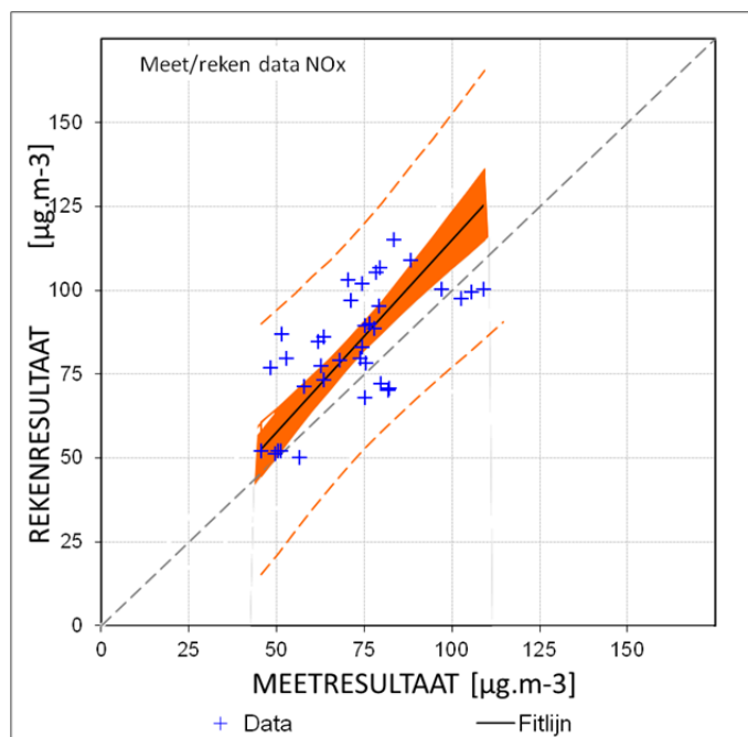
Figuur 5.6 Plot van gemeten en berekende \text{NO}_x -concentraties op straatstations in het LML (2009-2011) en het DCMR-metnet (2010-2011).
