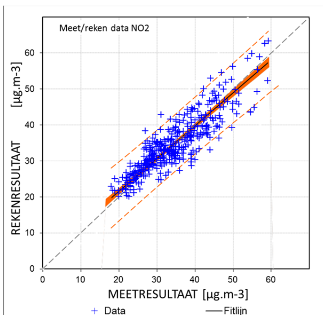
Figuur S1.4 Vergelijking van gemeten en met het RIVM-model voor 2010 en 2011 berekende NO 2 -concentratielocaties binnen het toepassingsgebied.
